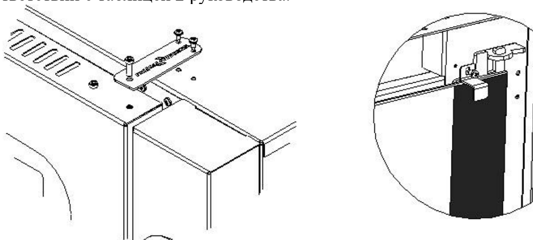
Рис.6 Транспортировочные крепления на двери ПР-04М, ПР-06М, ПР-10М.
