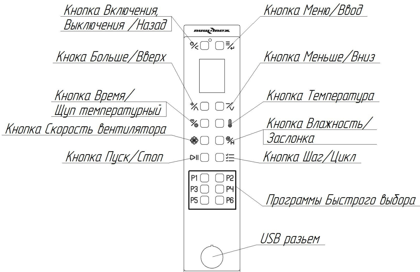
Рис.5 Внешний вид панели управления PR-DIW-06,PR-DIW-07, PPR-DIW-10,PR-DIW-12.
